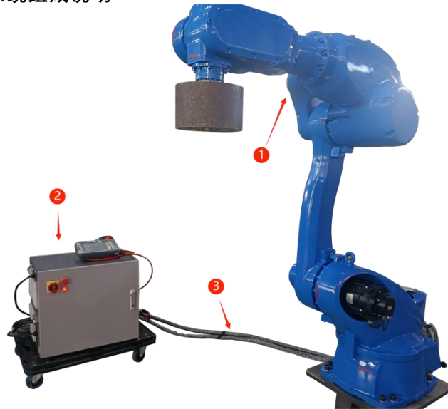
1——机器人本体；2——控制柜；3——连接线缆；
