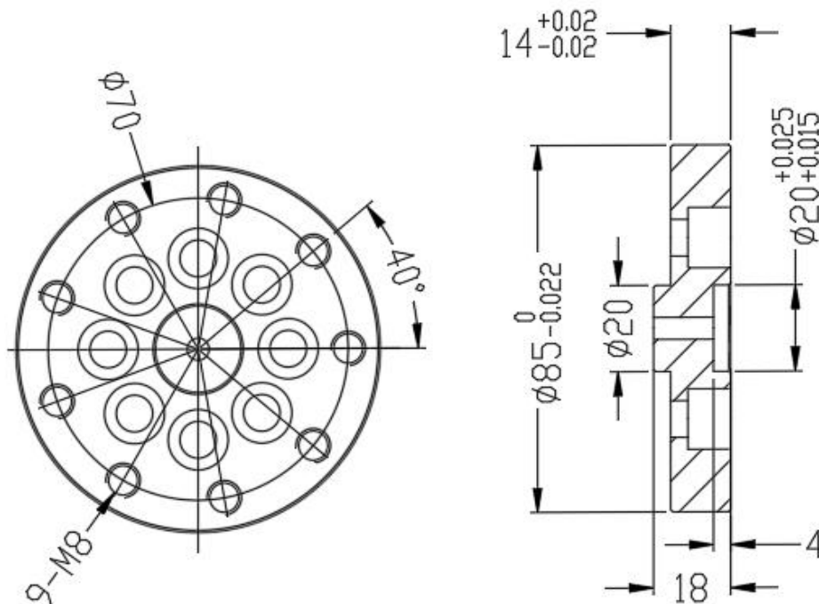
底座安装尺寸
