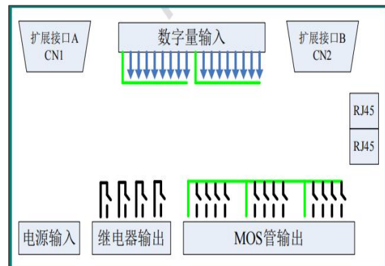
布局图
