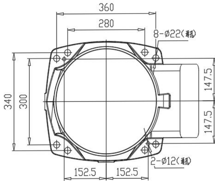
底座安装尺寸
