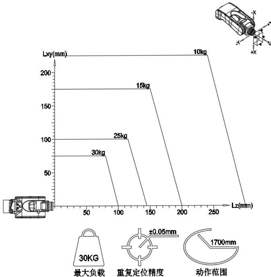
● MR30-1700 机器人腕部负载图
